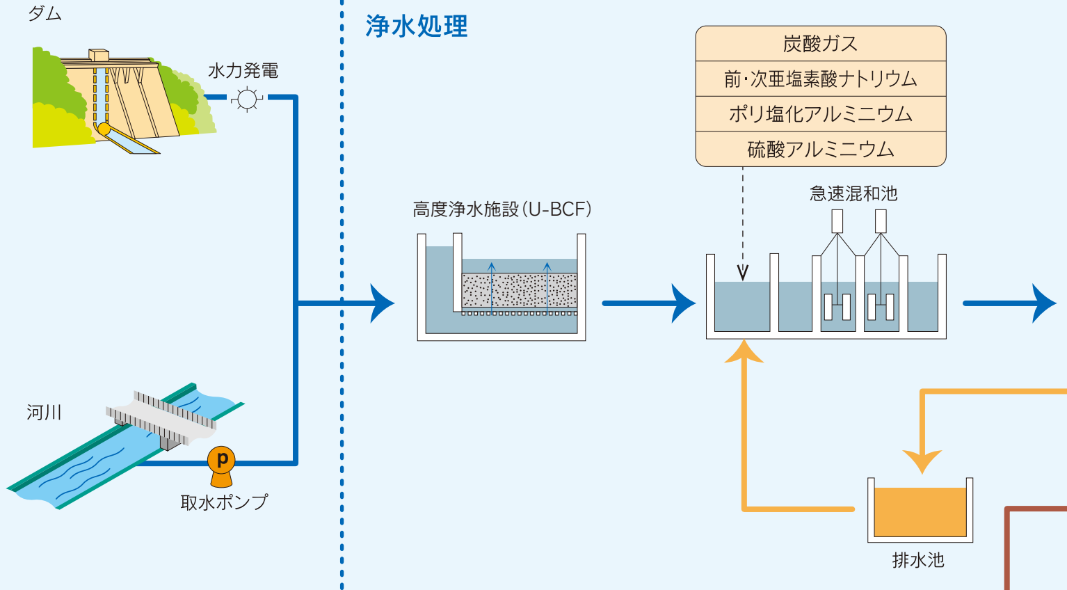
急速混和池
